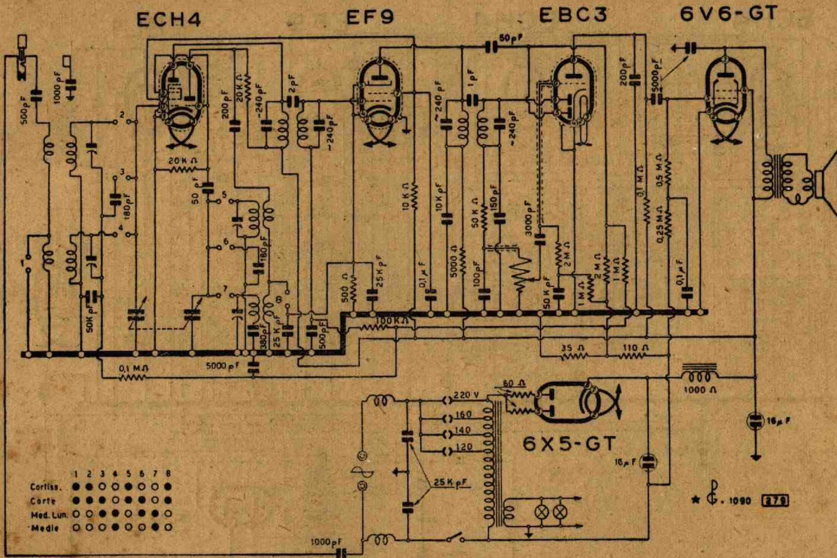
Lo schema elettrico del Phonola 573
